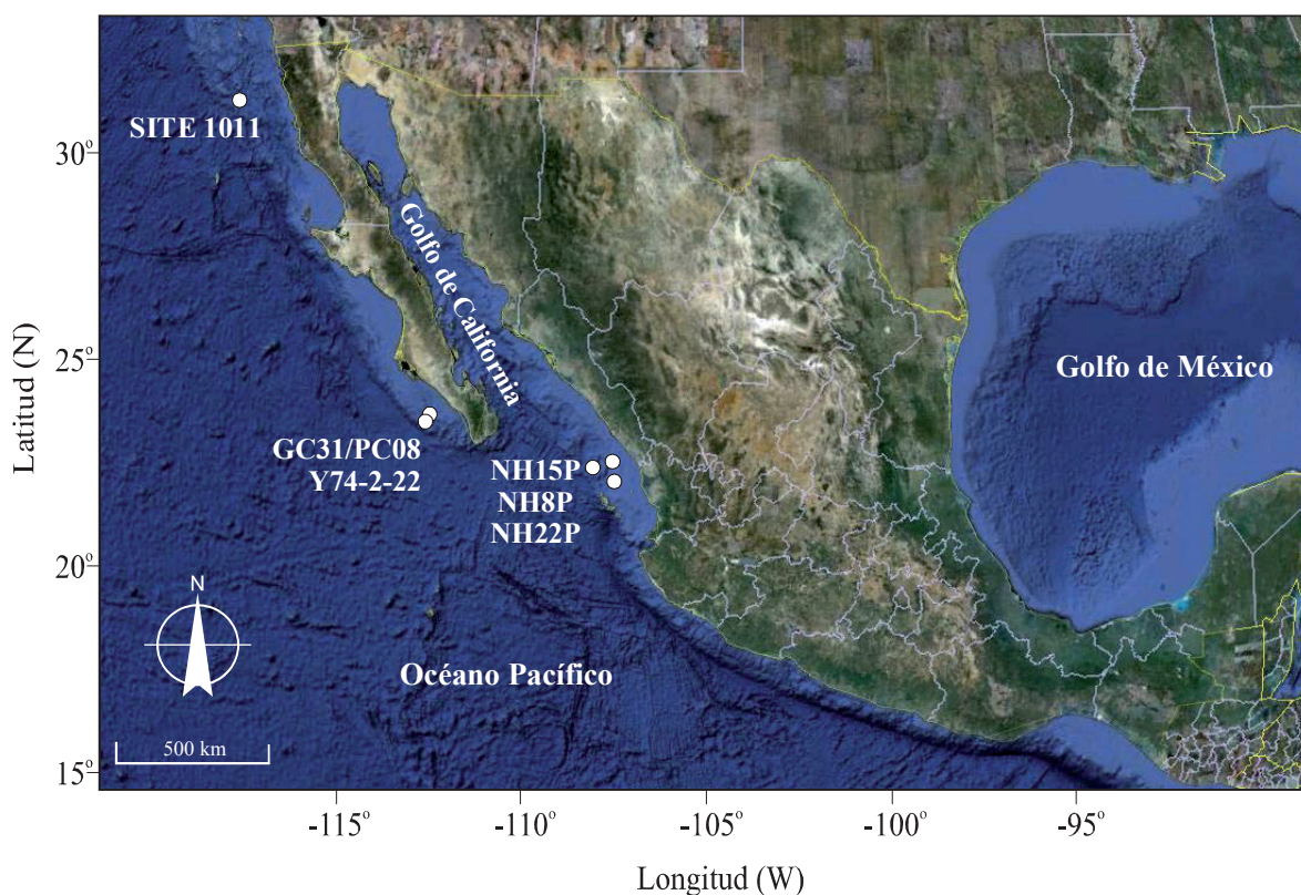
Figura 1. Localización de los sitios de colecta de los núcleos ODP167-SITE 1011 (Lyle et al. , 2000); GC31/PC08 (Sánchez y Carriquiry, 2007a, b); Y74-2-22 (Lyle et al. , 2000) y NH15P, 22P y 8P (Ganeshram y Pedersen, 1998) a lo largo del Pacífico oriental mexicano.
