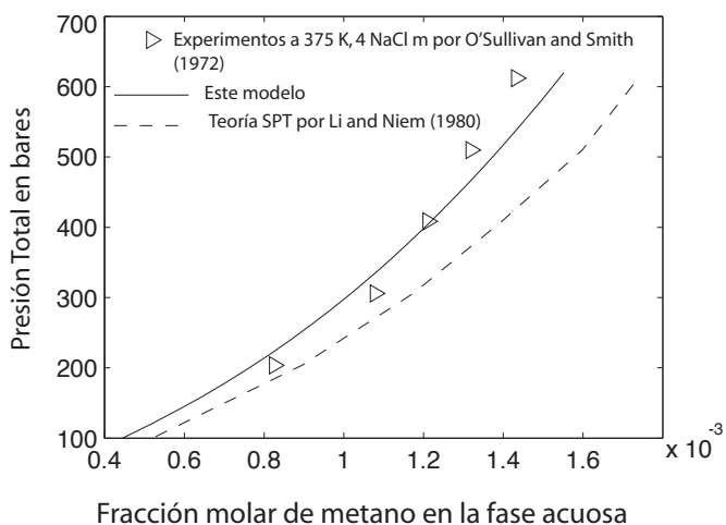
Figura 3. Datos experimentales y resultados de modelación de la solubilidad del metano a 375 K en una solución acuosa 4 NaCl molar.
